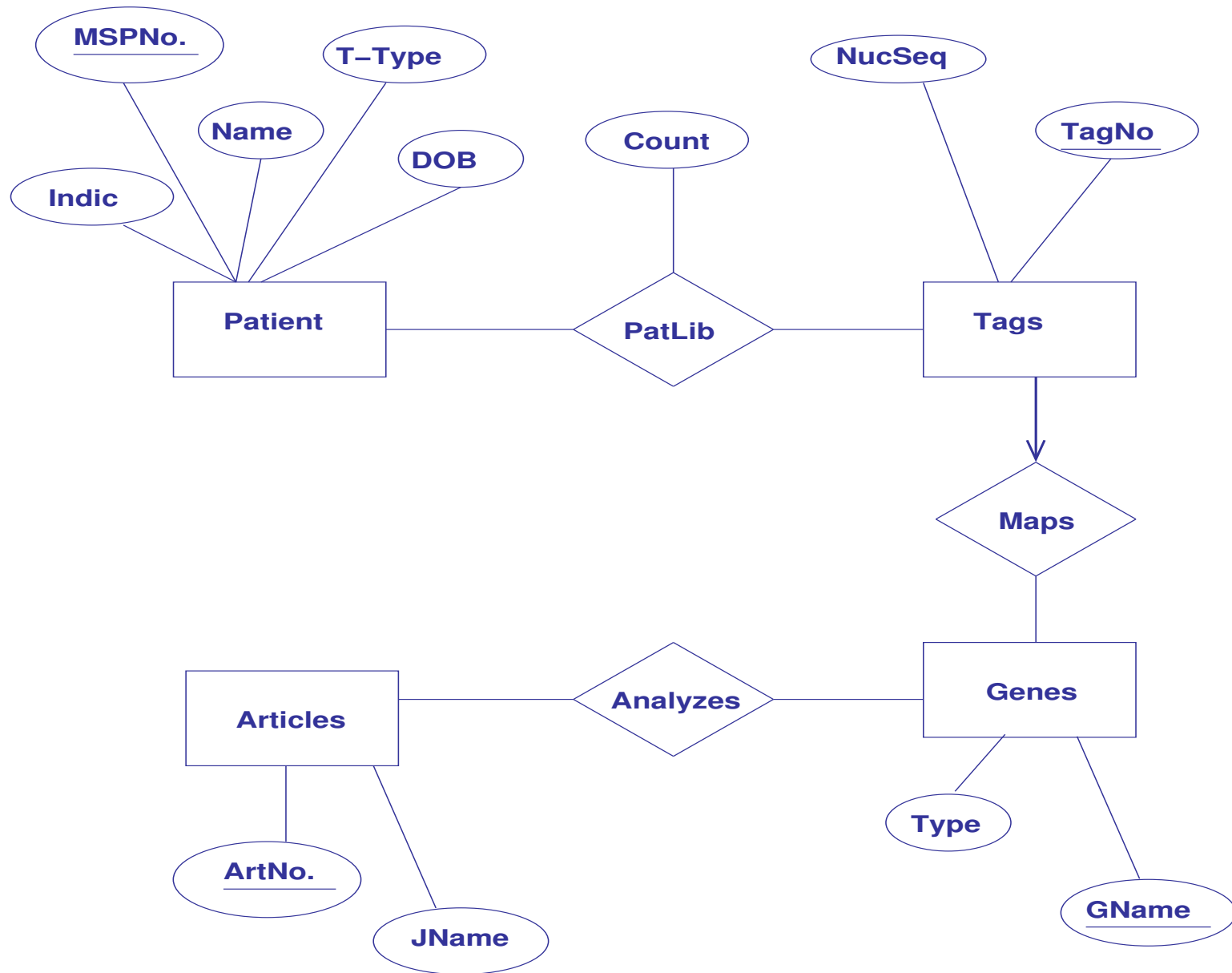
Figure 1: ER Diagram
