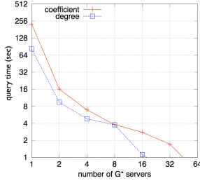
Fig. 29 Twitter speed up
