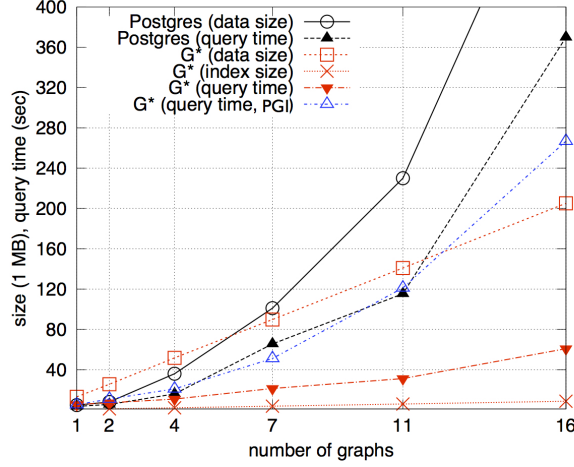
Fig. 20 G* vs PostgreSQL
