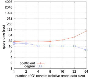
Fig. 26 Twitter scale up
